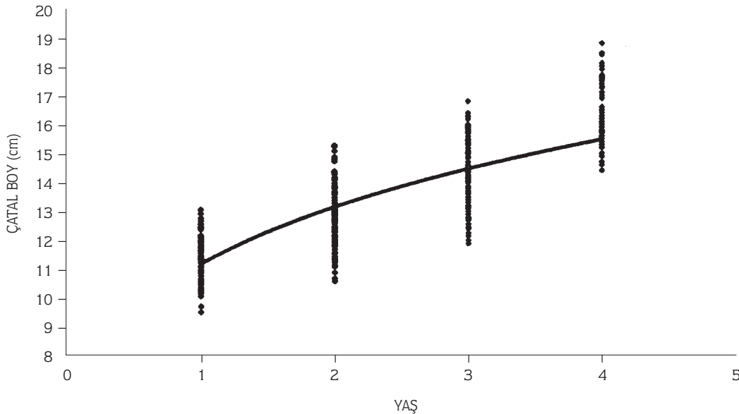
Şekil 2. Dişi+erkek M. barbatus bireylerinin yaş-boy ilişkisi eğrisi.
