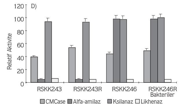
Şekil 2. Bifonksiyonel gene ait ksilanaz ve CMCse enzimleri için sıcaklık optimumu (A), pH optimumu (B), sıcaklık direnci (C), substrat seçiciliği (D) değerleri.
