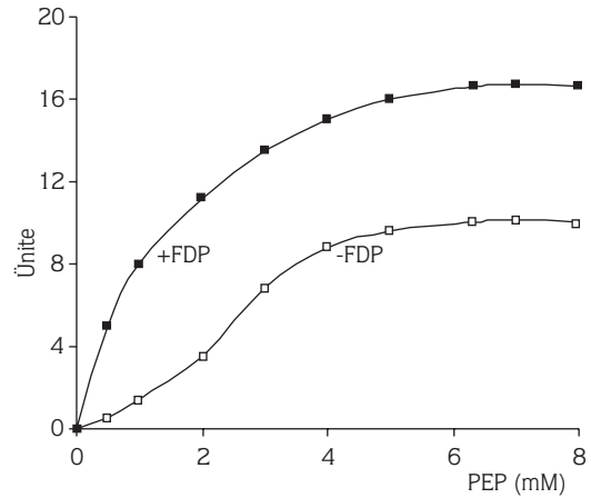
Şekil 10. Normal Rat Karaciğer Doku Pirüvat Kinaz Aktivitesinin PEP Konsantrasyonuna Bağlı Olarak Değişimi.
