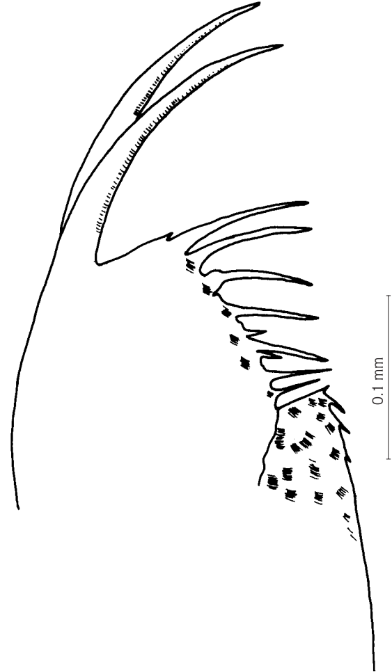
Şekil 3. Ceriodaphnia megops Sars, 1862 Postabdomen
