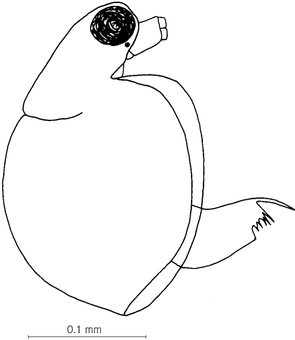
Şekil 2. Ceriodaphnia megops Sars, 1862 Genel görünüş.
