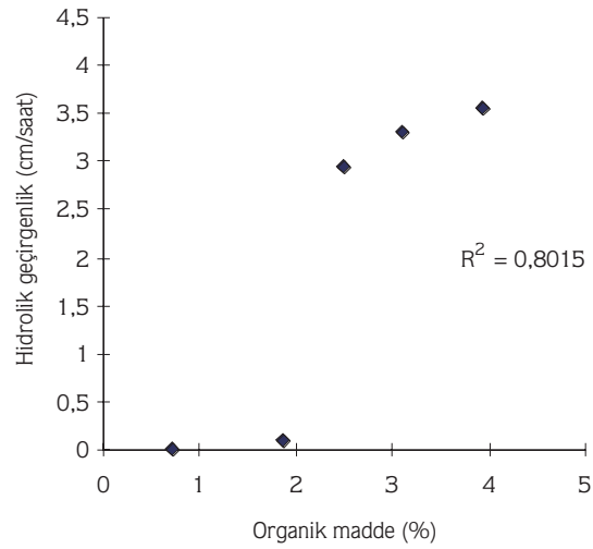
Şekil 2. Tütün tozu miktarına bağlı olarak hidrolik geçirgenliğin değişimi
